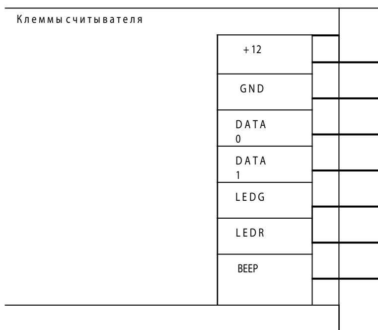
Рисунок 1. Клеммы считывателя «СЧИТ-АГРГ-ПОЛЯР»
